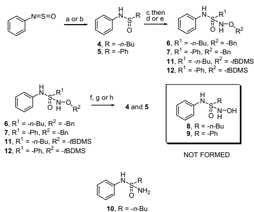
Scheme 2. Reagents: (a) n -BuLi; (b) PhMgBr; (c) t -BuOCl; (d) BnONH 2 ; (e) t -BDMSONH 2 ; (f) Pd/C, H 2 ; (g) TBAF; (h) CH 3 CO 2 H–H 2 O–THF.
